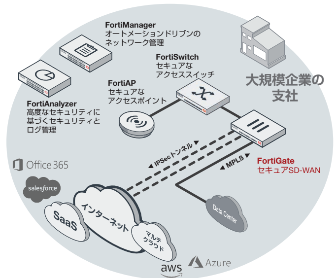
FortiGate 60F の大規模企業の支社への導入例 (セキュア SD-WAN)
