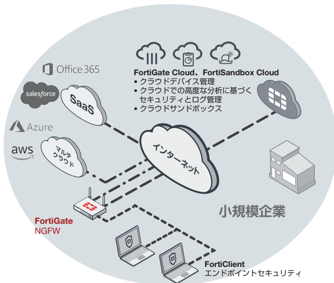
FortiWiFi 60F の小規模企業への導入例 (UTM)
